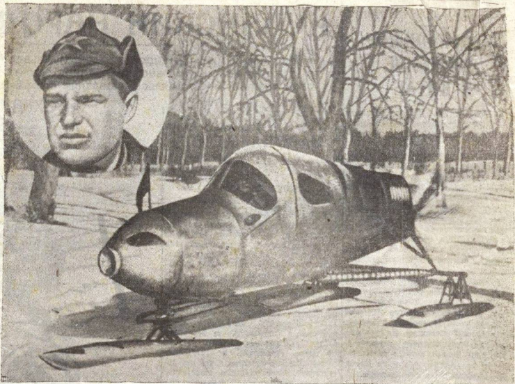
Аэросани с автомобильным мотором «ГАЗ», сконструированные и построенные начальником производства оренбургских механических мастерских т. Сафроновым. Сани развивают скорость до 60 км. в час. В овале тов. Сафронов.
